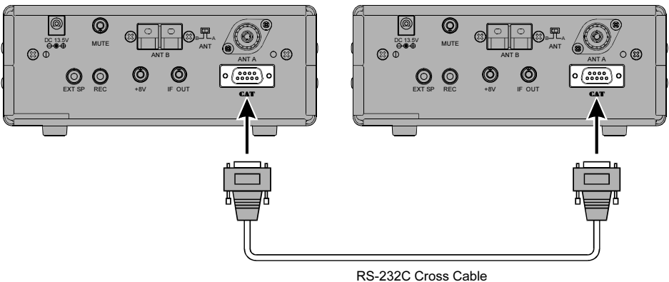
RS-232C Cross Cable
