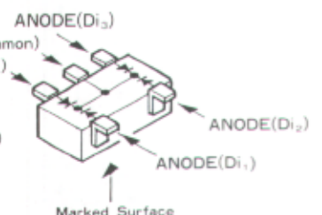
FMN1 (N1) (D204,205)
