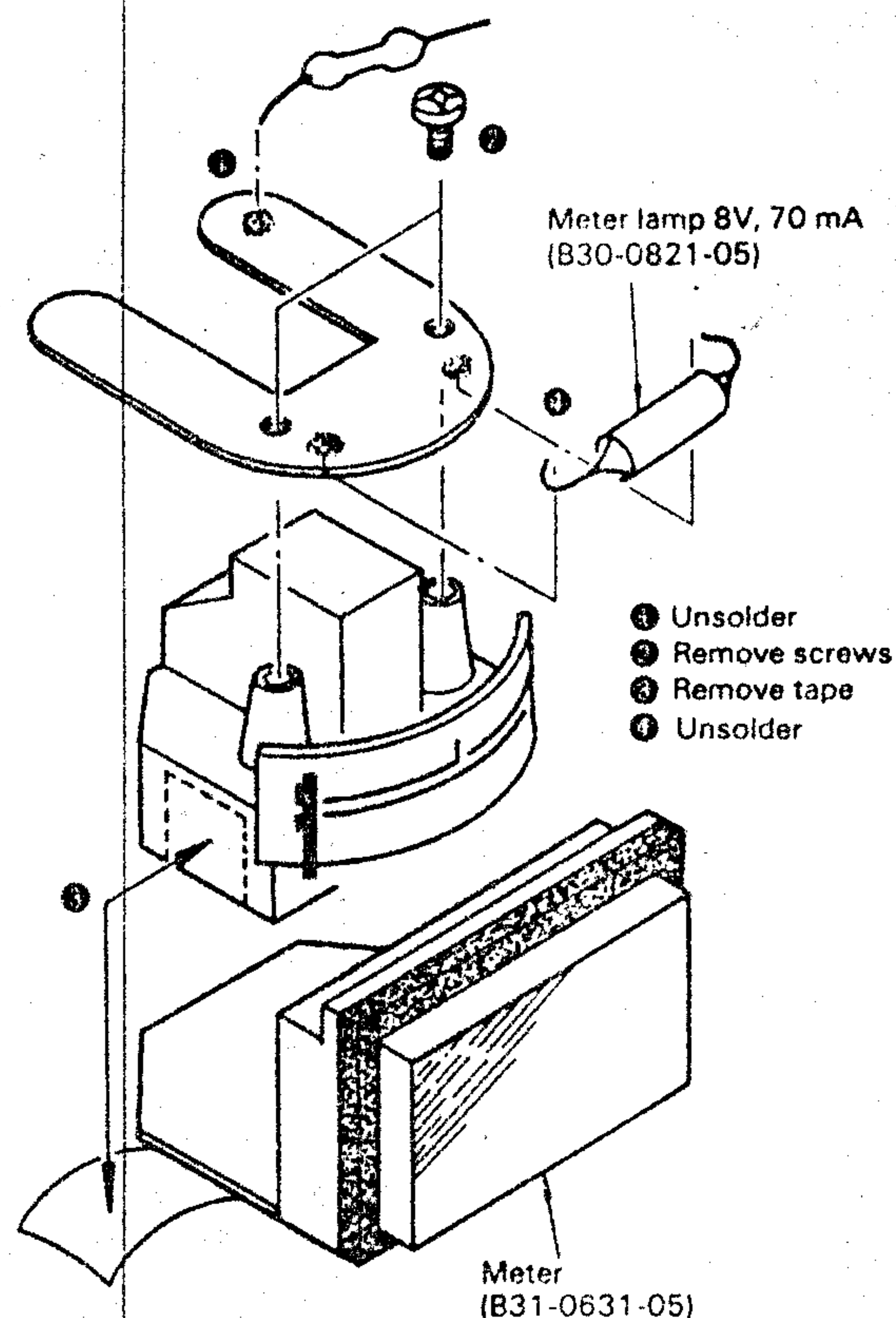
Fig. 17 Meter
