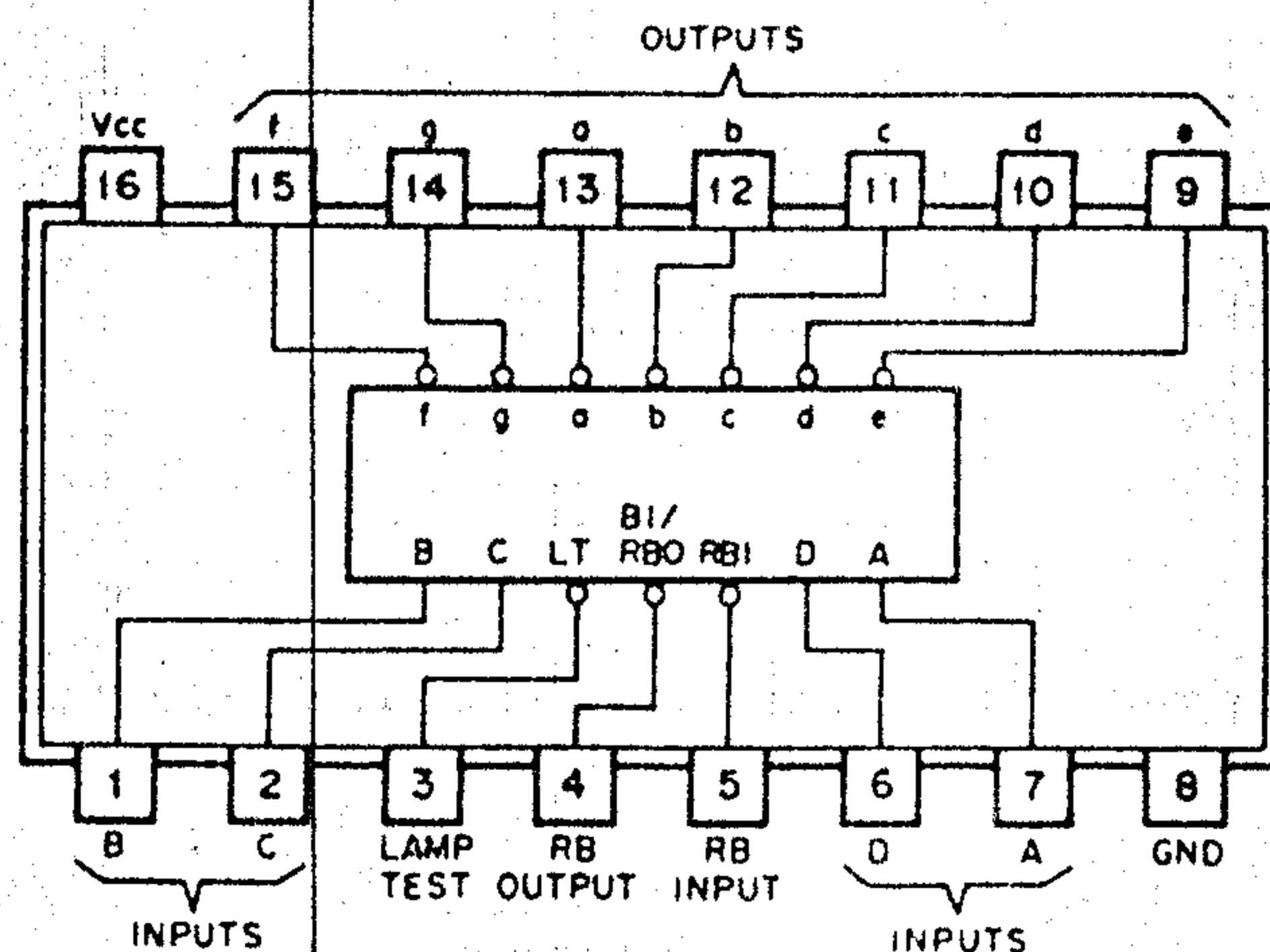
Fig. 8 SN74LS247N
