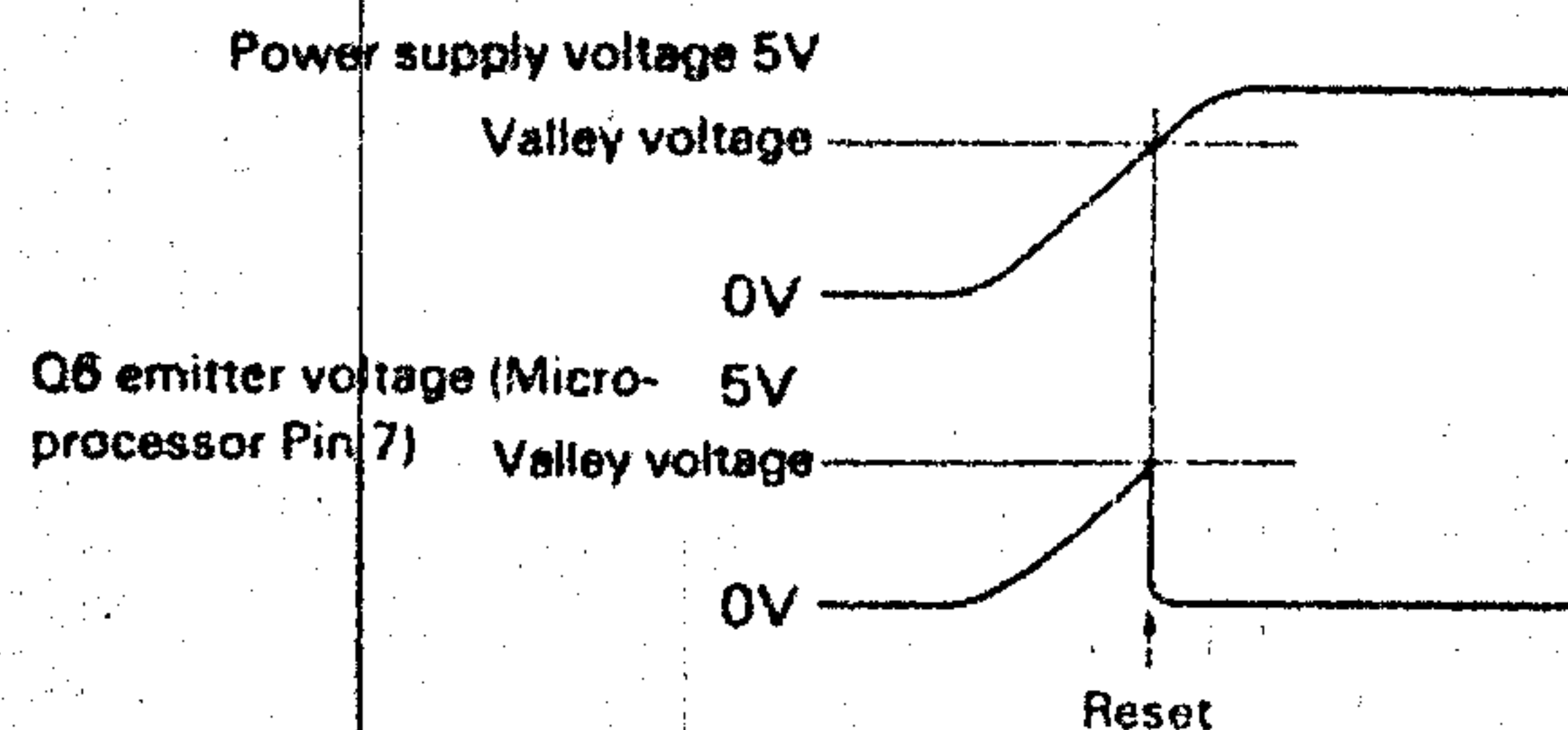
Fig. 11-A Reset timing
