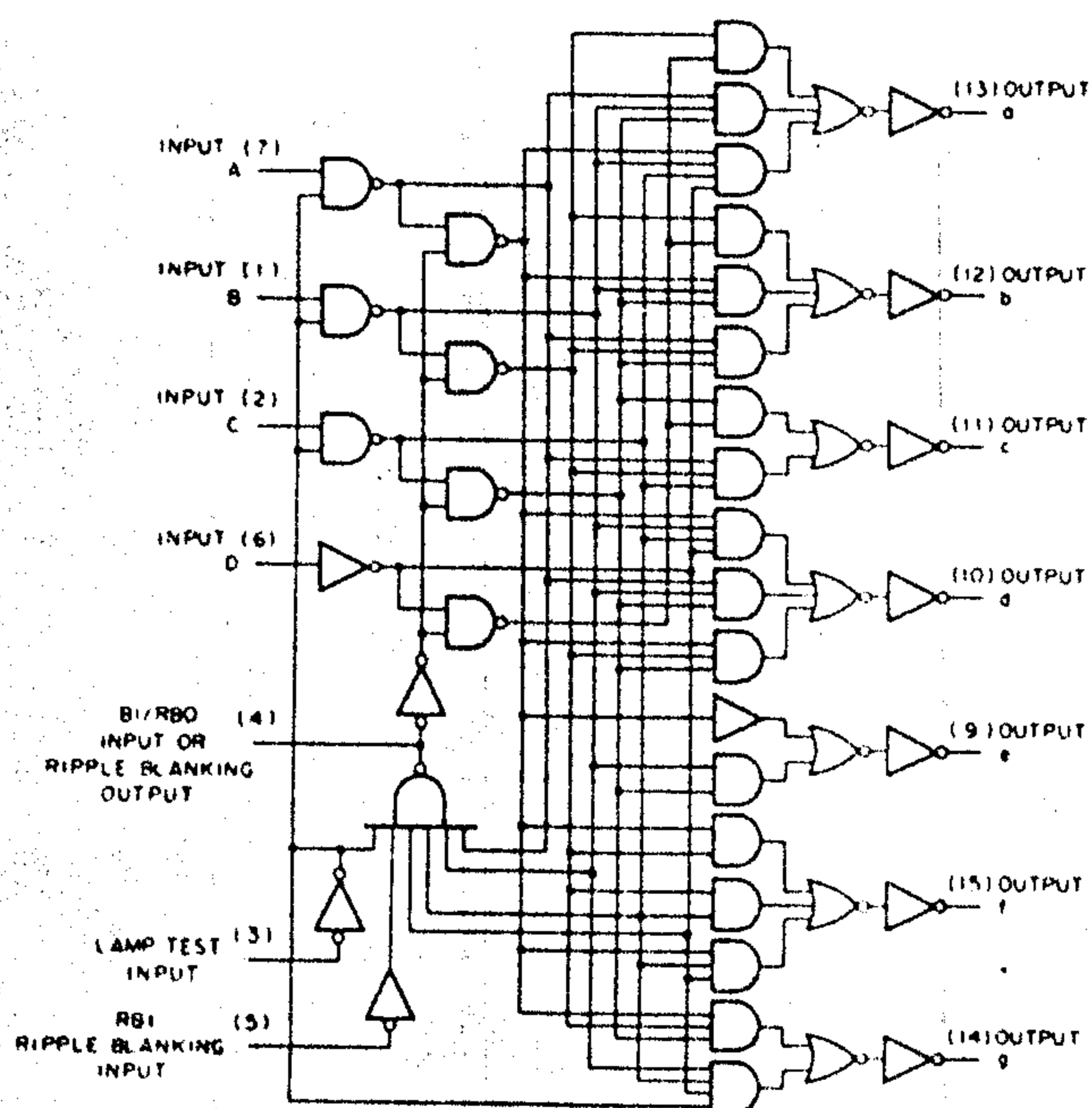
Fig. 7 SN74LS247N
